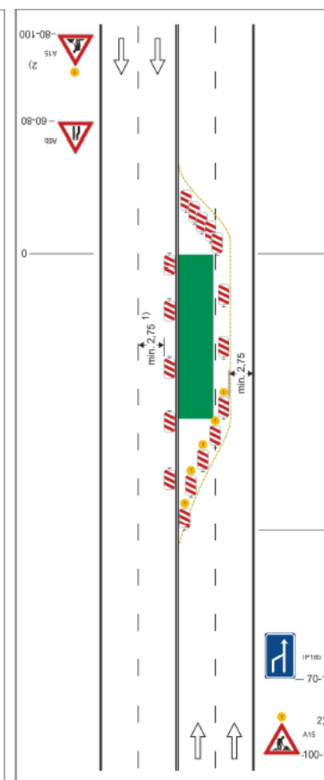
Schéma B/10
