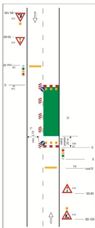
Schéma B/6
